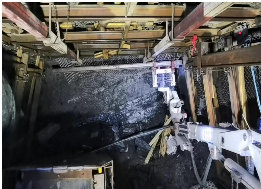
掘进工作面架棚机械手
