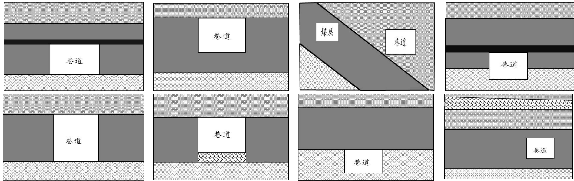
厚煤层巷道典型布置形式
