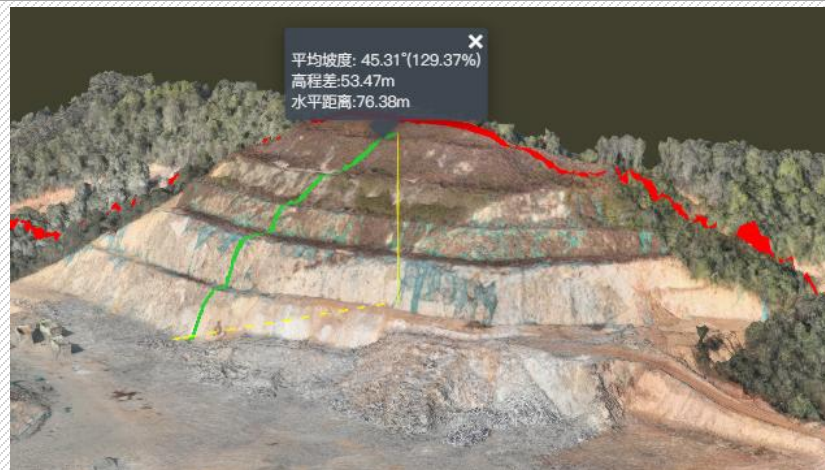
测坡角
